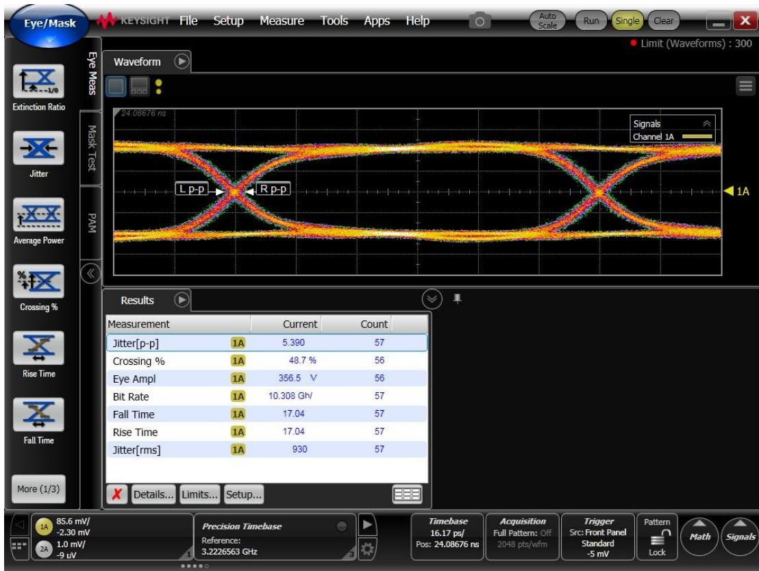
BERTWave E225A 设备 10.3125G、PRBS31 码型 眼图
