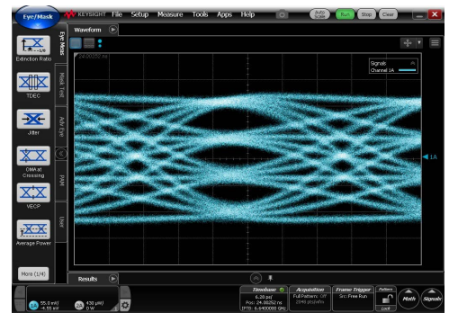
53.125 GBd 单端测试眼图
